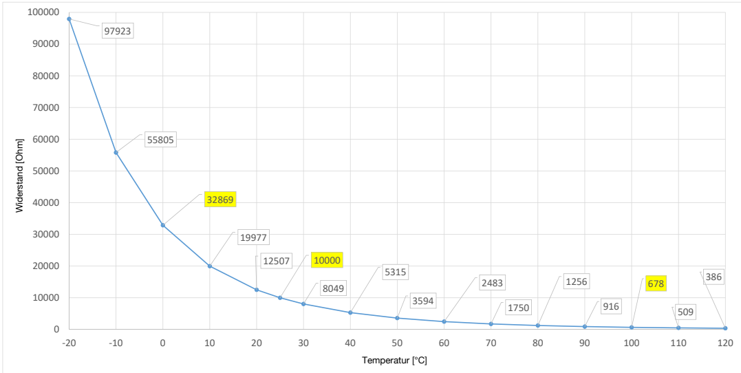
BEISPIEL EINER KURVE NTC 10Kohm B25/85= 3977K Example of curve NTC 10Kohm B25/85= 3977K
