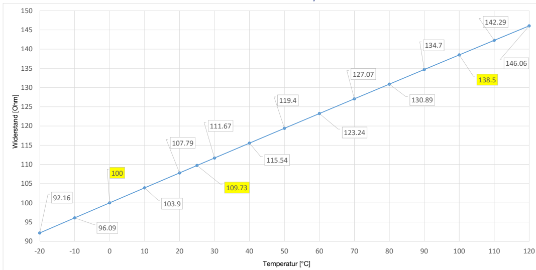
BEISPIEL EINER KURVE PT100 - IEC 751 Example of curve PT100 - IEC 751
