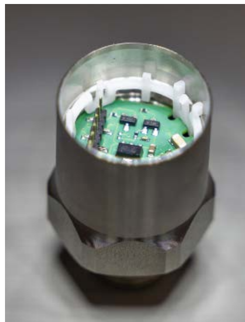
Sopra. Sensore assemblato; Il dettaglio interno testimonia il rigore nella fase di ingegnerizzazione
